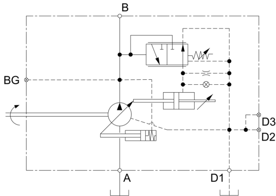
C0 Schematic
